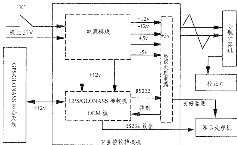
图 2 双卫星定位校正系统的组成框图
